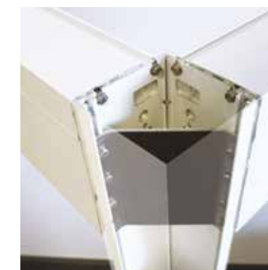
Gepatenteerde hoekversterking in de palen voor een muurvaste, onwrikbare constructie
